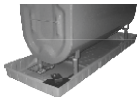
Plateau large pour nouveaux réservoirs d'acier pour 200 et 250 gallons
